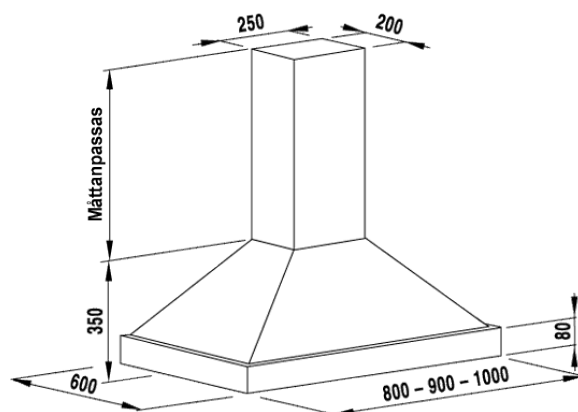
Måttskiss
