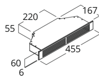
Kanalgällersats
