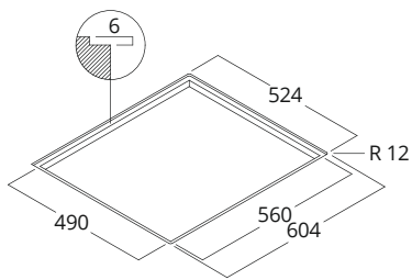
Infälld montering
