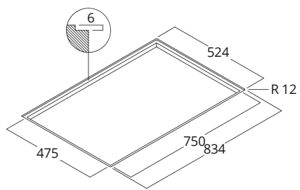
Infälld montering
