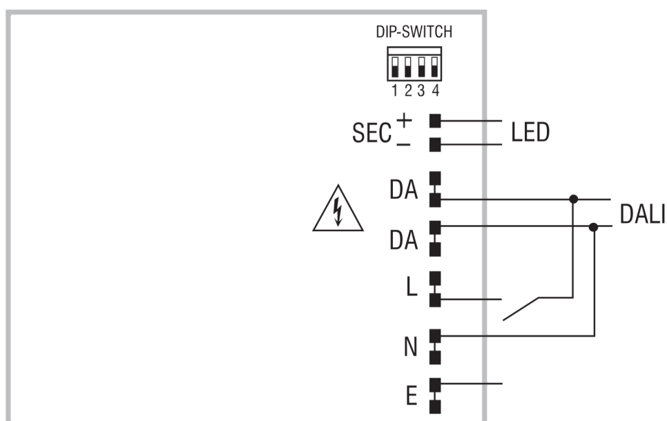
PUSH SWITCH diagram - Inkopplingsanvisning EL
