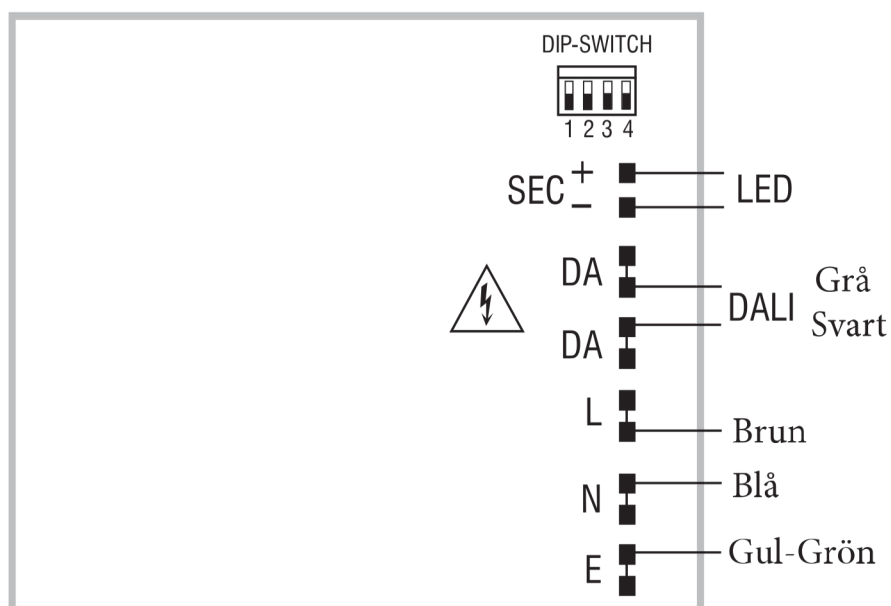
DALI diagram - Inkopplingsanvisning El
