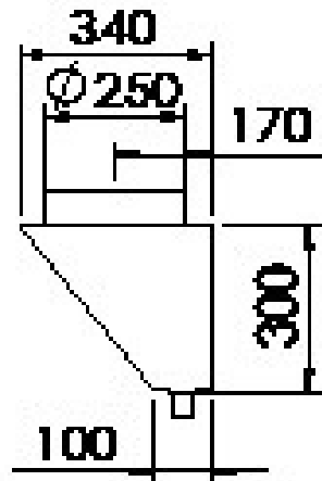
FHV 5025 (väggfilterhus)
