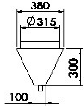
FHC 5025 (centrumfilterhus)
