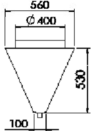
FHC 5050 (centrumfilterhus)
