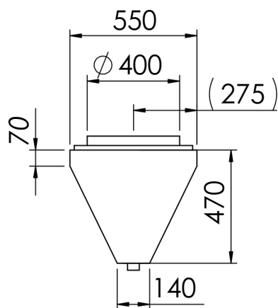
Centrumfilterhus
