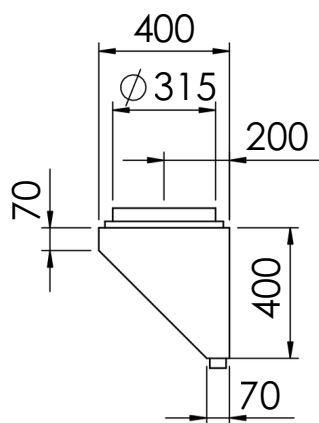
Väggfilterhus
