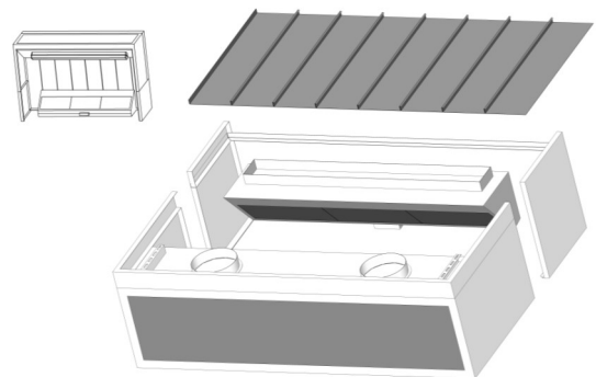
CJ kåpa
