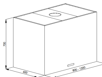
Måttskiss
