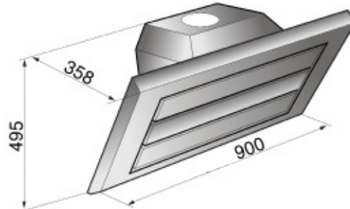
Version md Cupolino, tillbehör vid kolfilterdrift för ersättning av standardkanal
